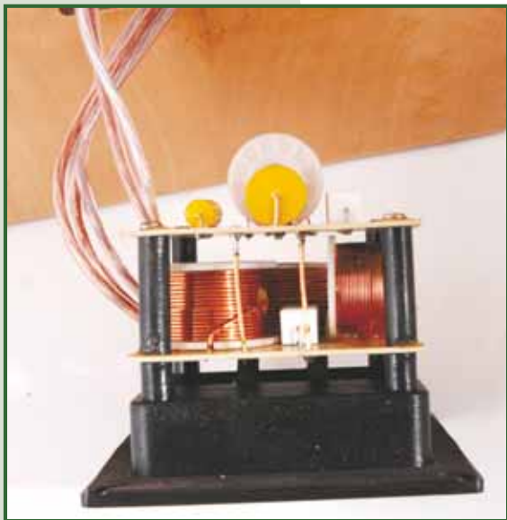
Il complesso delle induttanze.
